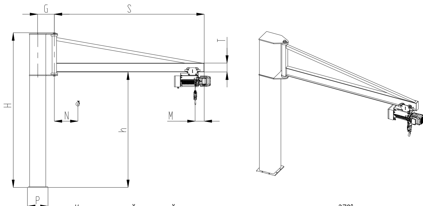
Кран консольный с оттяжкой с ручным поворотом стрелы- угол поворота 270°
